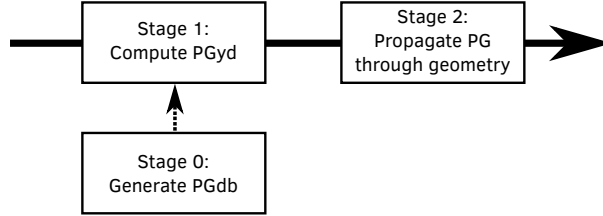
Figure A.14: Flow chart de la méthode vpgTLE. L'étape 0 est une base de données PG initiale (PGdb) et est calculée une fois. Chaque simulation subséquente est divisée en étape 1 et étape 2. L'étape 1 génère une distribution de rendement PG spécifique au CT (PGyd) en utilisant un nombre limité de primaires. Dans l'étape 2, PGyd est utilisé pour générer et propager un ensemble représentatif de PG dans toute la géométrie.
