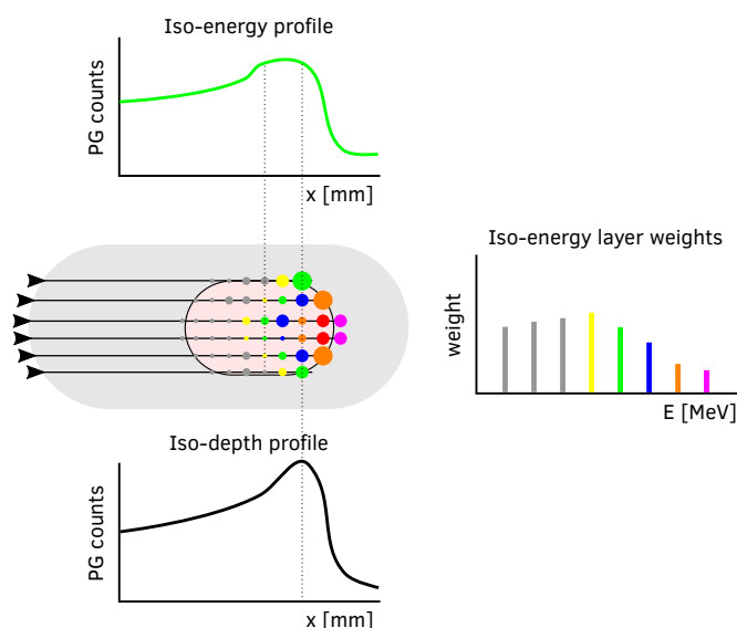
Figure A.22: Une vue schématisée d'un patient (gris clair), d'un volume de traitement planifié (rose-pêche) et d'un faisceau de protons (lignes horizontales noires venant de gauche). Superposés sont des taches variées, où la taille des cercles indique des poids ponctuels. Les couleurs ponctuelles indiquent la couche d'iso-énergie dont le spot fait partie. À droite, les poids (comptage de protons) par couche iso-énergie sont tracés. En haut, le profil PG est esquissé pour une couche iso-énergie. En bas, le profil PG est esquissé pour la couche iso-depth (spots de différentes couleurs sur la ligne pointillée). En violet et en rouge, les quatre points sur l'extrémité distale des deux lignes de faisceau les plus centrales, l'effet de l'interpolation est illustré: chaque position distale n'est pas toujours prévue avec un poids élevé.
