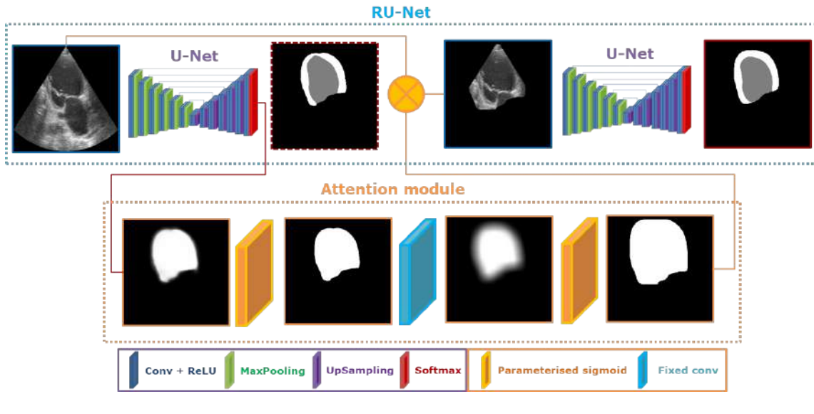
FIGURE 1.10: Illustration du modèle RU-Net. Les deux U-Nets sont indépendants (paramètres séparés).
