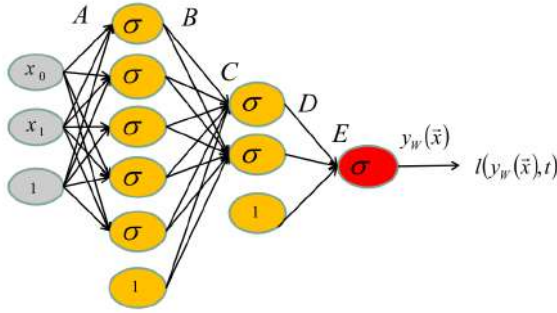
(a) Illustration de rétropropagation sur un réseau neuronal entièrement connecté [36]
