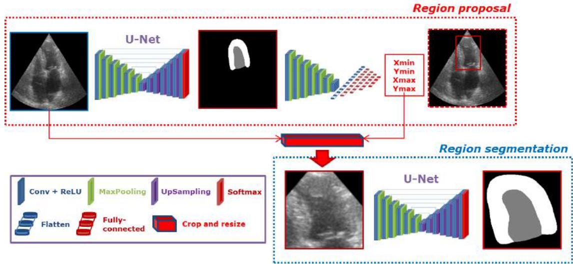
FIGURE 1.11: Illustration du modèle LU-Net avec le réseau de proposition de région U-Loc2-multi-région, décrit dans la section 9.5.1. Les deux U-Nets sont indépendants.
