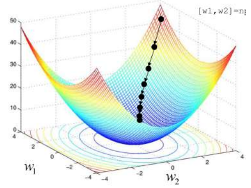
(b) Paysage d'optimisation : convergence itérative depuis une initialisation aléatoire [36]
