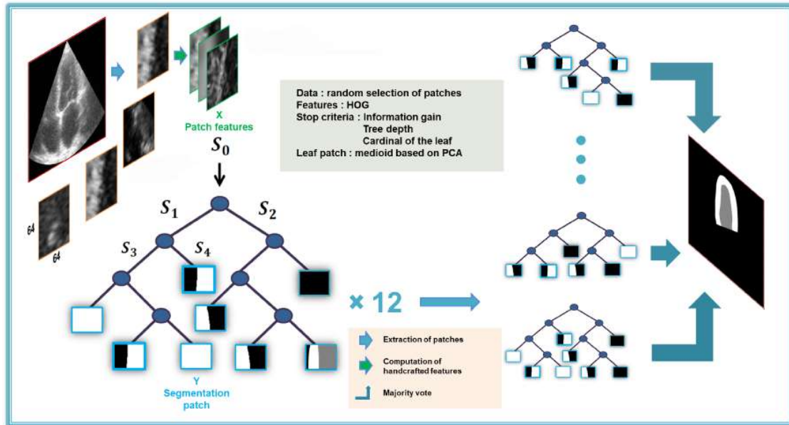
FIGURE 1.6: Notre méthode SRF [31]
