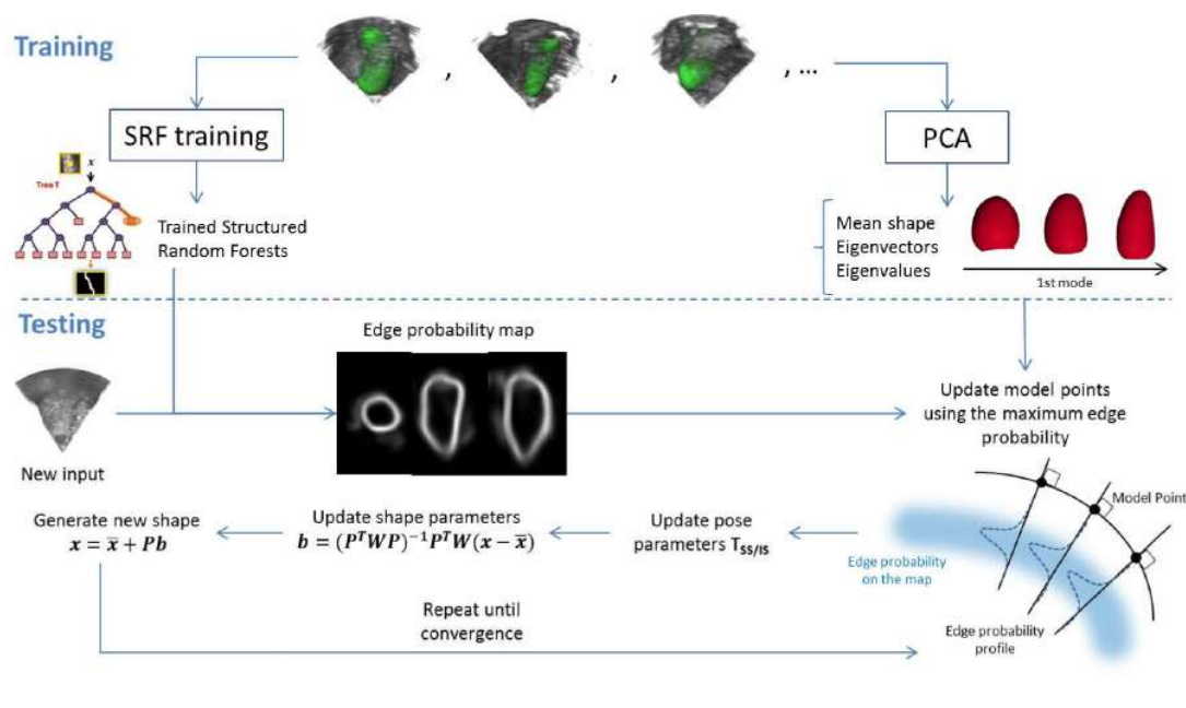
FIGURE 1.7: Vue d'ensemble de notre pipeline complet combinant SRF et ASM pour la segmentation du ventricule gauche en échocardiographie 3D.
