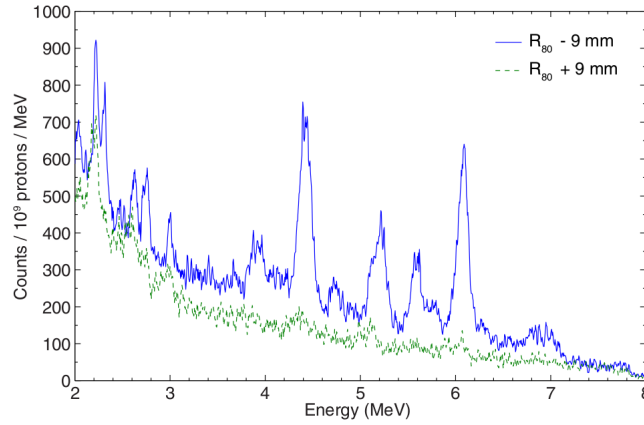
FIGURE 6.8 – Spectre énergétique du rayonnement gamma-prompt intégré sur une fenêtre temporelle de 2 ns, mesuré 9 mm avant et 9 mm derrière la fin du parcours notée R_{80} (figure extraite de [90]).
