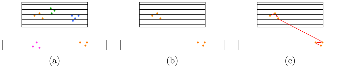
FIGURE 5.5 – Création des événements à partir des interactions dans MEGALib. Chaque photon est suivi individuellement (pas de coïncidences aléatoires) et ses interactions sont représenté avec la même couleur (a). Les photons ayant touché seulement le diffuseur ou seulement l'absorbeur sont écartés. Pour un photon donné (b), l'ordre des interactions est inconnue pour Revan et déterminée par un algorithme (c). Dans la séquence ainsi ordonnée on retient les positions des deux premiers points ainsi que l'énergie déposée lors de la première diffusion et la somme des énergies déposées par la suite.
