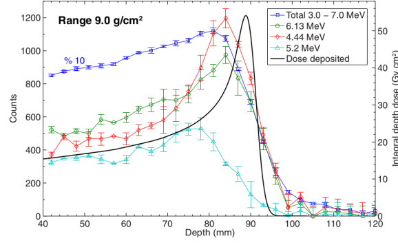
FIGURE 6.10 – Distribution en profondeur des émissions gamma-prompt cumulé et discrètes comparées au profil de dose (ligne noire) (figure extraite de [90]).
