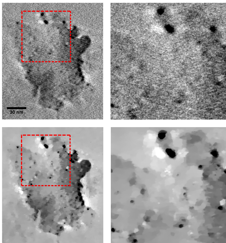
FIGURE 7.6 – Reconstruction d'un échantillon \text{Pd}/\text{Al}_2\text{O}_3 avec SIRT (ligne en haut) et SIRT-FISTA-TV (ligne en bas). Une coupe XY de chaque volume reconstruit est montrée dans la première colonne et un agrandissement de la région marquée par un rectangle rouge est montré dans la seconde colonne.
