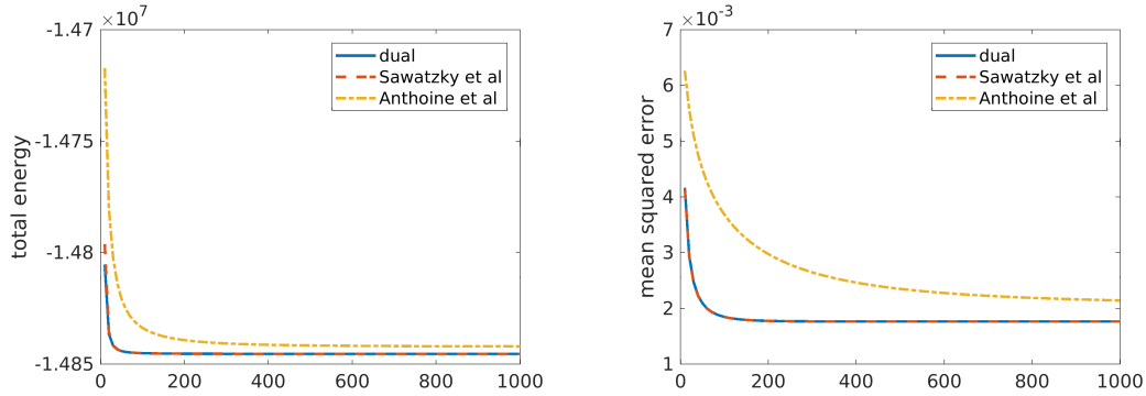
FIGURE 6.16 – Comparaison en termes de minimisation du critère et de l'erreur quadratique moyenne entre la méthode duale proposée (ligne bleue), la méthode de Swatzky et al [65] (ligne rouge) et celle de Anthoine et al. [5] (ligne jaune).
