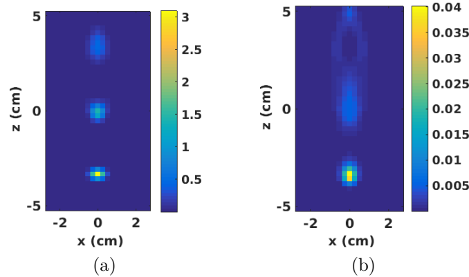
FIGURE 6.17 – Image reconstruite avec l'algorithme MLEM à partir de projections avec (a) une erreur de 2.5^\circ sur l'inclinaison de l'axe \alpha et (b) une erreur de 2.5^\circ sur l'angle de diffusion Compton \beta . Dans les deux cas, vingt itérations ont été effectuées.
