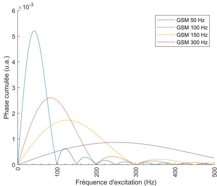
Figure 10. Phase cumulée (en unité arbitraire) pendant l'application d'un cycle gradient sinusoïdal de 50, 100, 150, 300 Hz selon la fréquence d'excitation.
