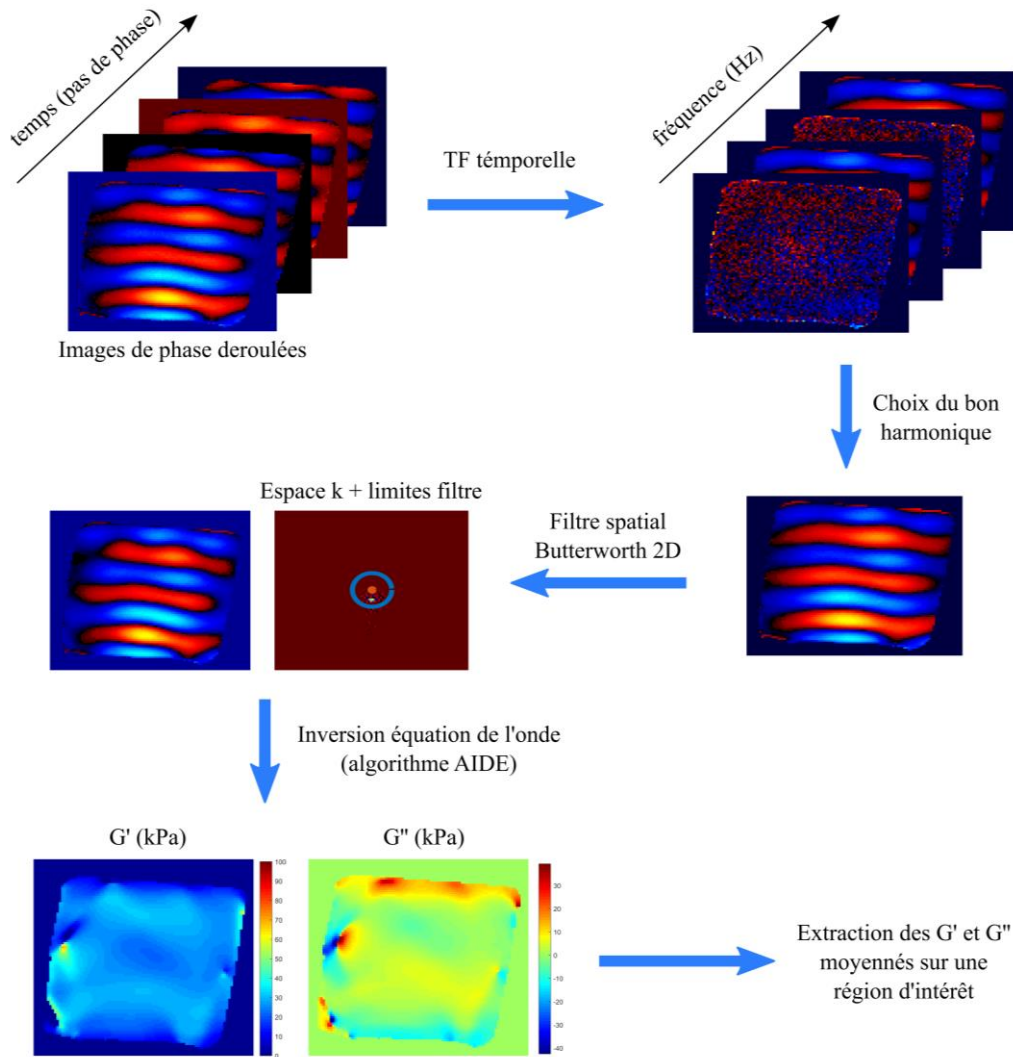
Figure 9. Schéma qui résume les étapes suivies dans cette thèse pour la reconstruction des données ERM jusqu'à l'obtention des valeurs moyennes du module de conservation et de perte de cisaillement
