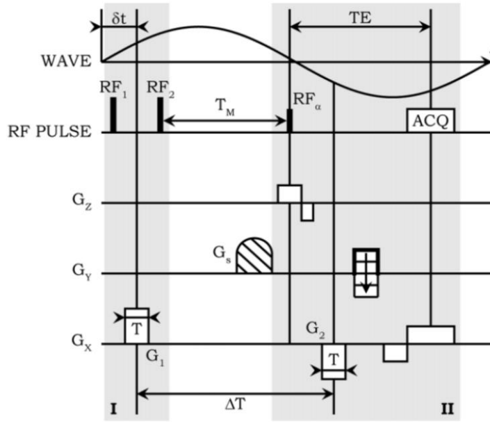
Figure 11. Chronogramme séquence DENSE (figure extraite de Robert et al. 11 )
