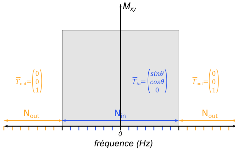
Figure 13. Définition du problème de contrôle optimal dans le cas d'une impulsion RF sélective. N_{in} et N_{out} correspondent aux isochromats considérés au sein et en dehors de la coupe, respectivement. T_{in} et T_{out} sont les états cibles fixés par l'utilisateur.
