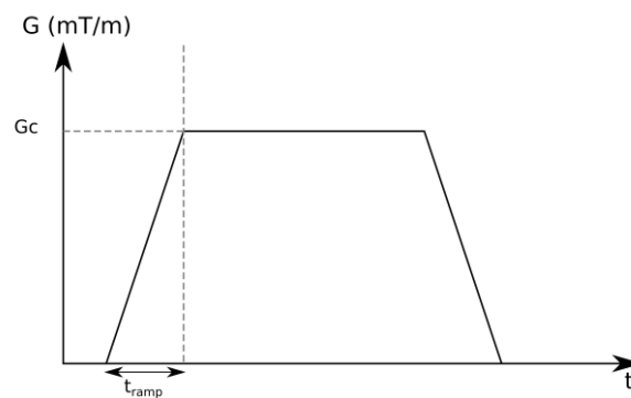
Figure 3. Représentation de l'application d'un gradient de champ magnétique sur un chronogramme de séquence
