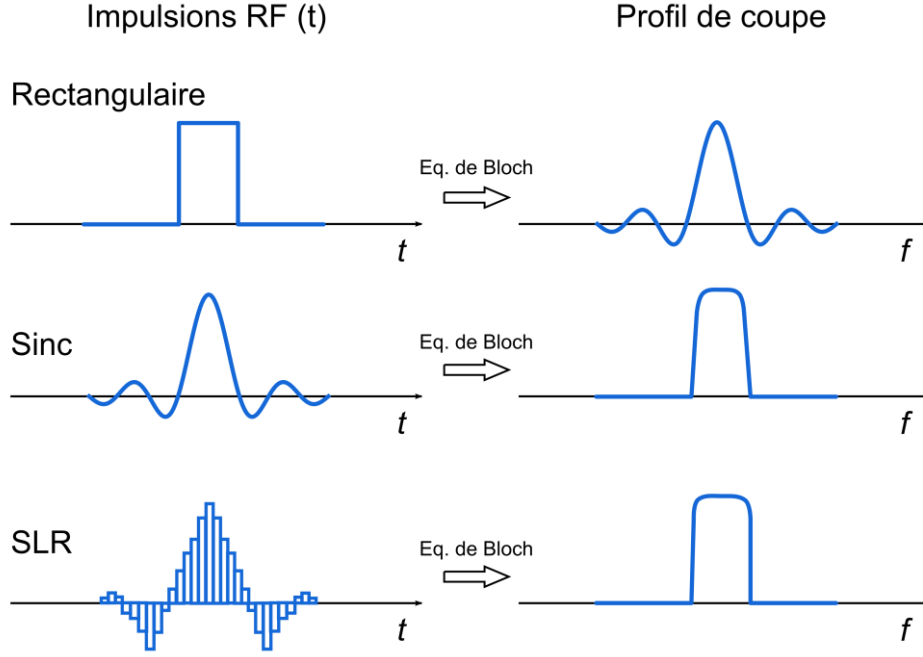
Figure 12. Illustration des différentes formes d'impulsions RF : A gauche, évolution temporelle de l'amplitude des impulsions; à droite : réponse fréquentielle correspondante.
