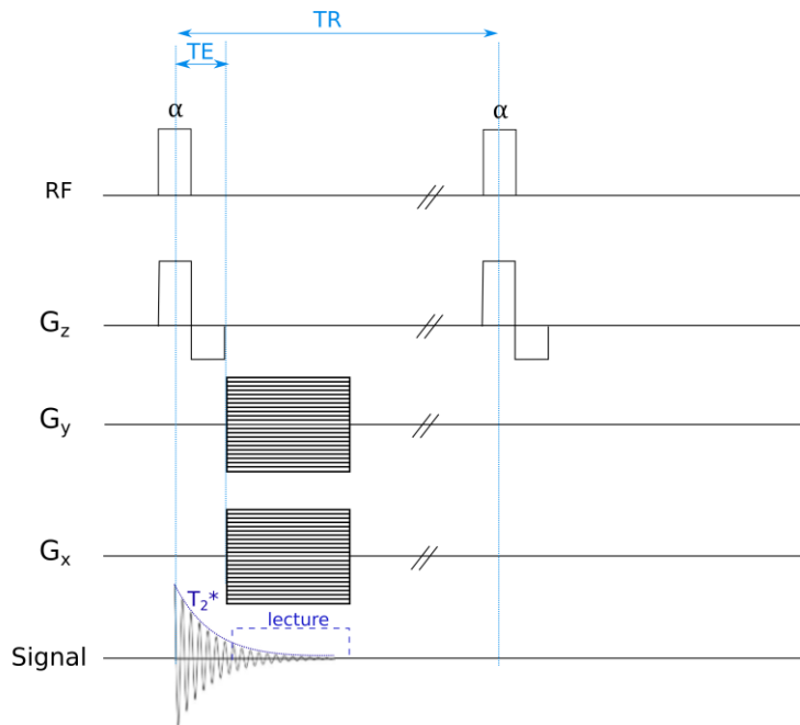
Figure 5. Chronogramme d'une séquence UTE
