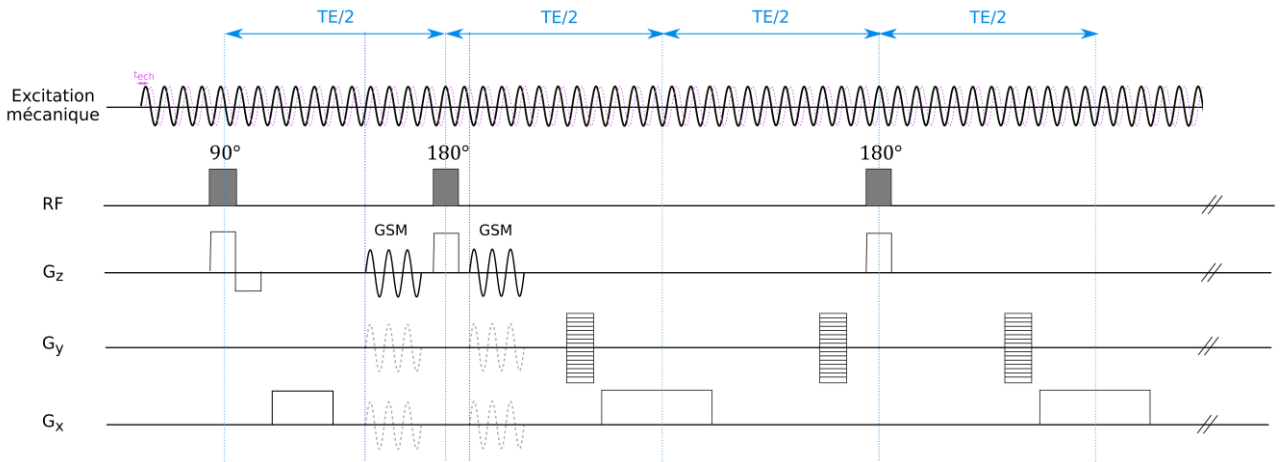
Figure 7. Chronogramme de la séquence ERM écho de spin rapide (RARE) utilisée pendant la thèse
