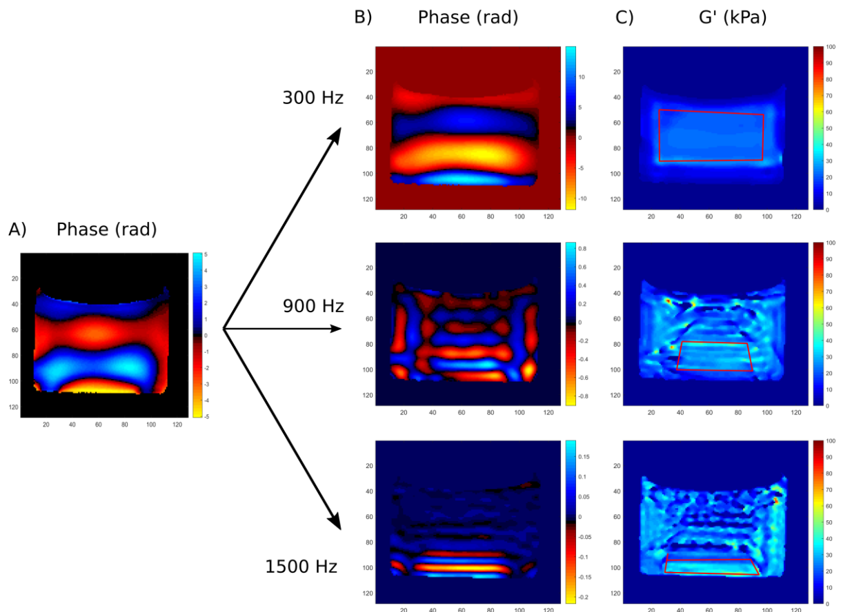
Figure 22. A) Image de phase de l'excitation tri-fréquence (rad). B) Images de phase (rad) et C) élastogrammes G' (kPa) de chaque composante fréquentielle extraite : 300 Hz en haut, 900 Hz au milieu et 1500 Hz en bas. La ROI utilisée pour le calcul de la moyenne et des écarts types du module de conservation est représentée par des lignes rouges sur les cartographies de la colonne C.
