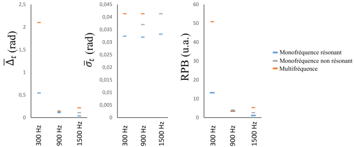
Figure 24. Comparaison des acquisitions mono et multifréquence à chaque fréquence en termes de phase encodée, bruit de phase et rapport phase sur bruit.
