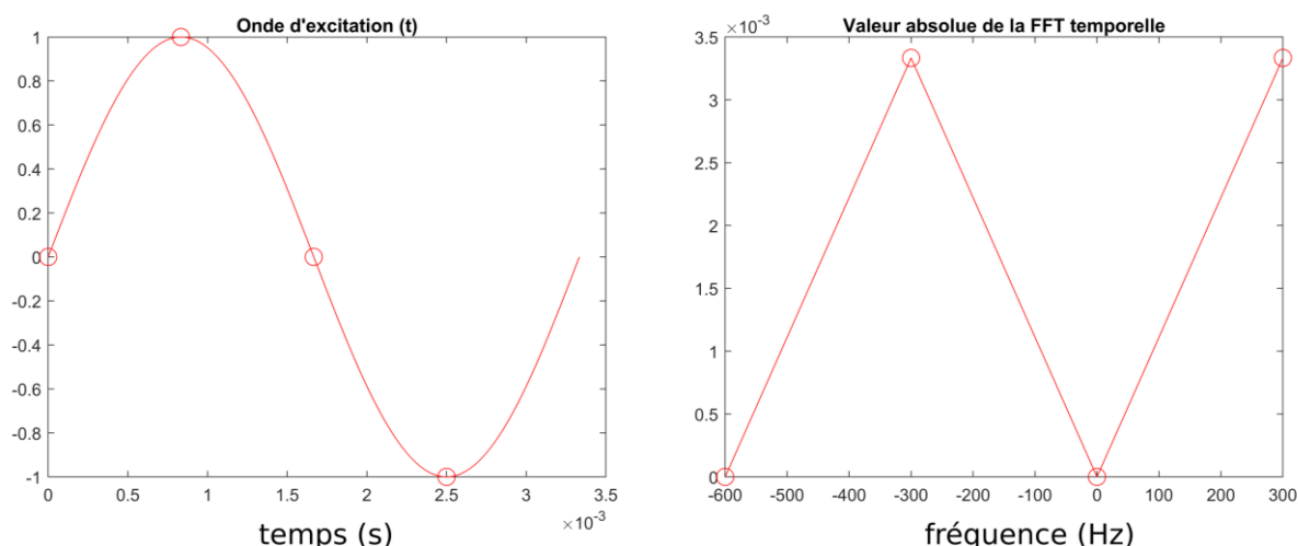
Figure 8. A gauche : points échantillonnés avec 4 pas de phase pour une onde de 300 Hz. A droite : après application de la transformée de Fourier temporelle, on obtient un premier harmonique à 300 Hz.
