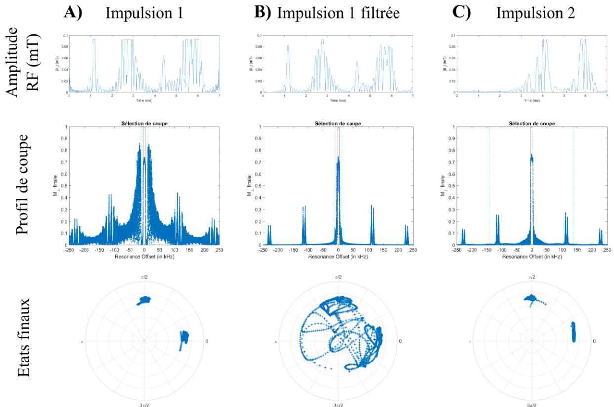
Figure 36. Amplitude des impulsions CO, amplitude de l'aimantation transverse des isochromats pour la plage fréquentielle [-250, 250] kHz et états finaux des isochromats se trouvant dans la coupe. Les lignes roses et vertes correspondent aux limites de la bande passante et les bandes extérieures dans les figures des profils de coupe.
