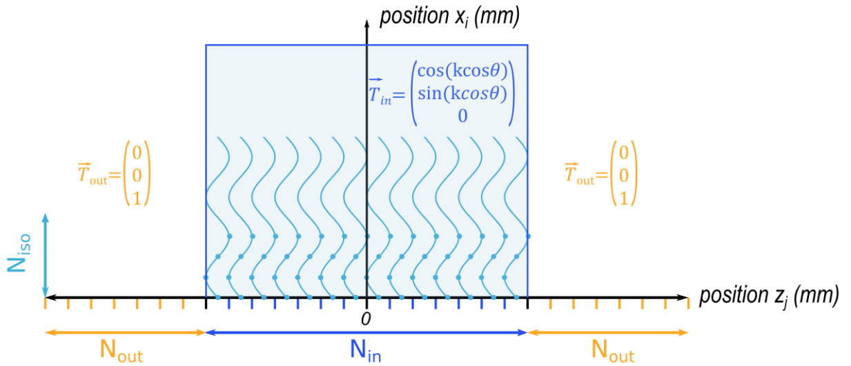
Figure 14. Définition du problème de contrôle optimal dans le cas de l'ERM. N_{in} et N_{out} correspondent aux isochromats considérés à l'intérieur et en dehors de la coupe, respectivement. \vec{T}_{in} et \vec{T}_{out} sont les états cibles fixés par l'utilisateur. N_{iso} correspond aux isochromats discrétisés le long d'une longueur d'onde de l'excitation mécanique (indiqués avec des points).
