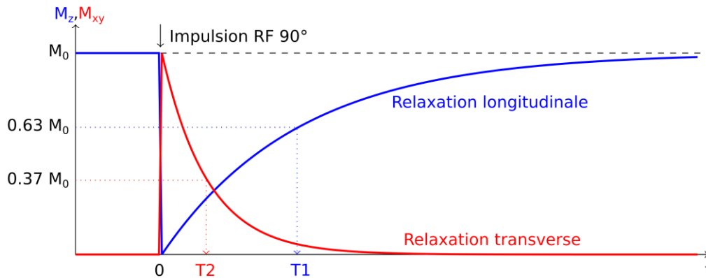
Figure 2. Evolution temporelle des aimantations longitudinale et transverse après une impulsion d'excitation de 90^\circ .
