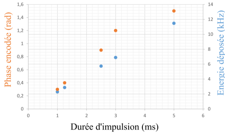
Figure 37. Phase encodée (en orange) et énergie déposée (en bleu) de chaque impulsion optimisée pour des durées différentes
