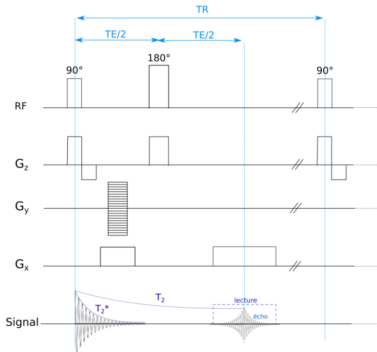
Figure 4. Chronogramme d'une séquence d'écho de spin
