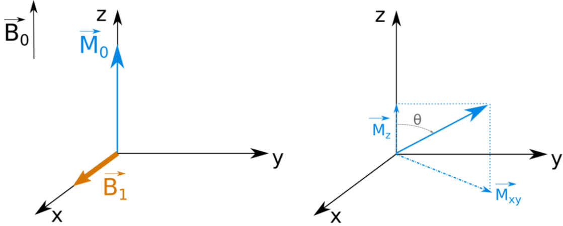
Figure 1. A gauche : l'impulsion d'excitation \vec{B}_1 est appliquée dans une direction perpendiculaire à \vec{B}_0 . A droite : l'aimantation est ensuite basculée d'un angle \theta donné.
