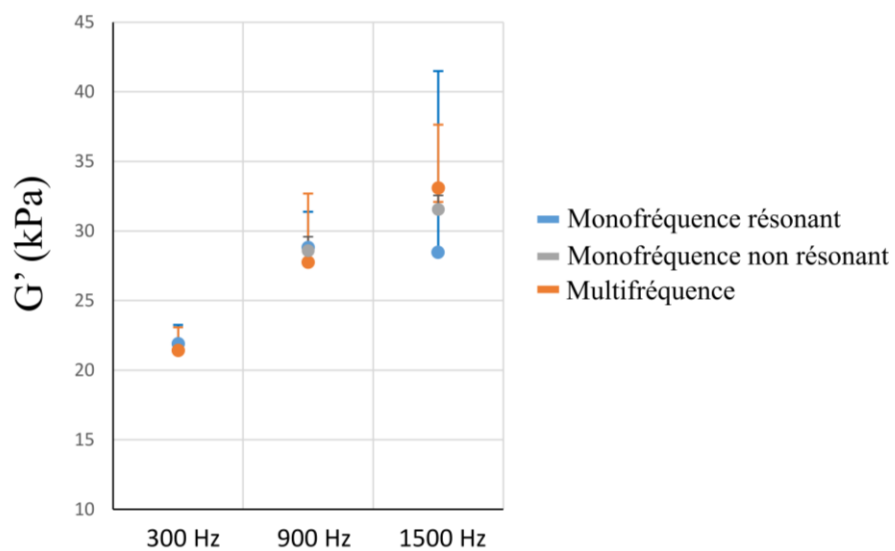
Figure 23. Valeurs moyennes, avec les déviations standard affichées sous forme de barres d'erreur positives, du module de conservation aux trois fréquences considérées avec les différents modes d'acquisition.
